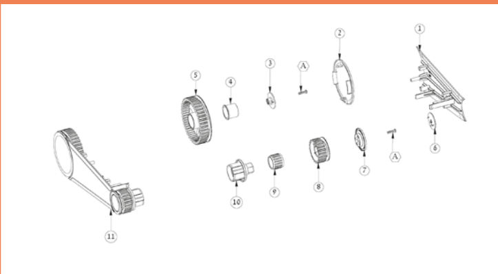
Ingranaggi spazzole - 40
