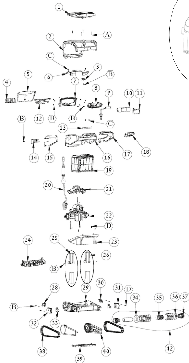
Ingranaggi spazzole - 40
